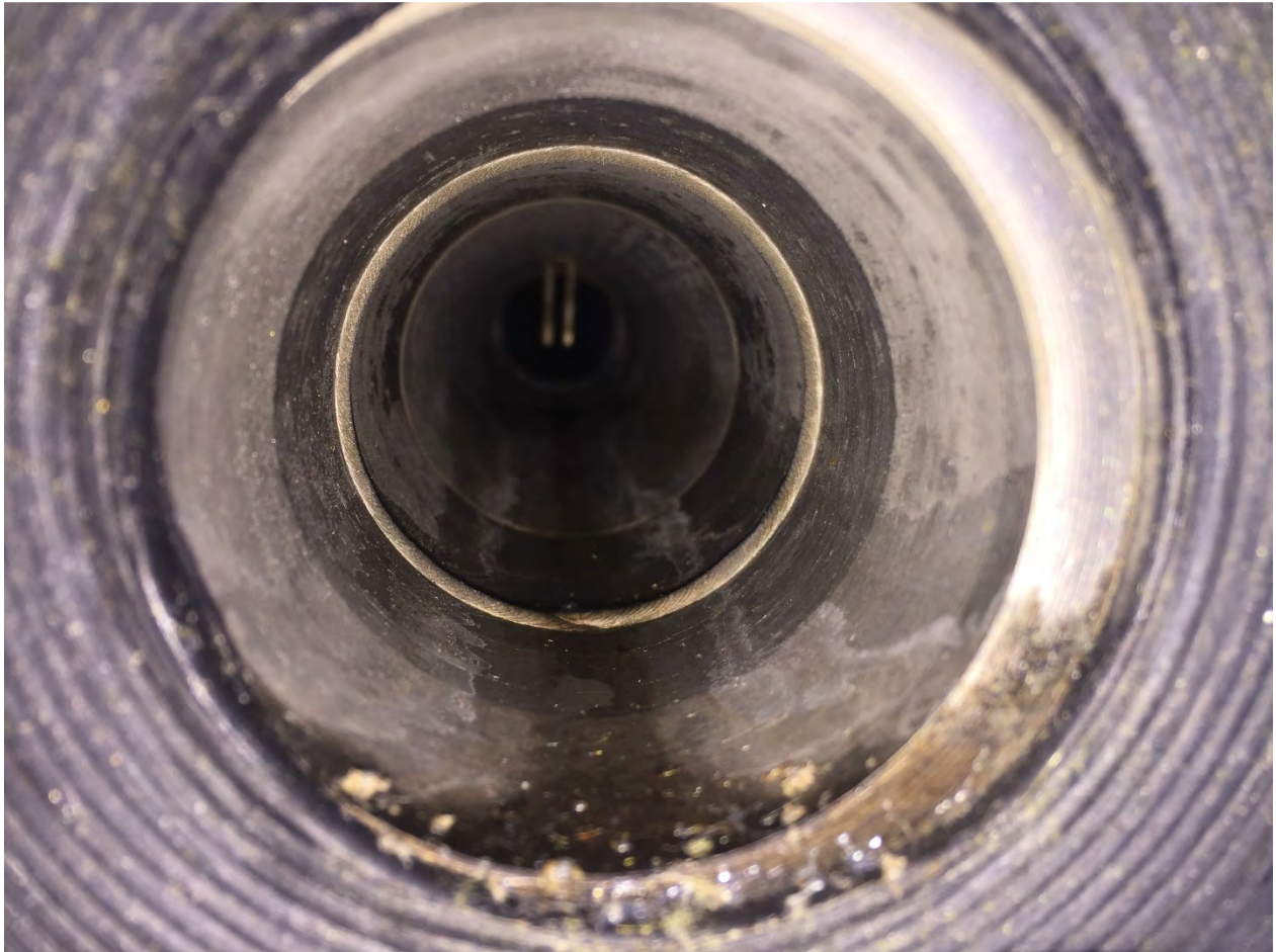
Photo du débitmètre de la RIDR (LET) lors de l'inspection du 25 octobre 2017
