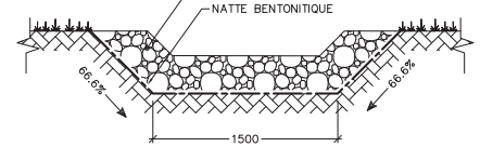
DÉTAIL TIPIQUE FOSSE EN BAS DE TALUS Echelle: Aucune
