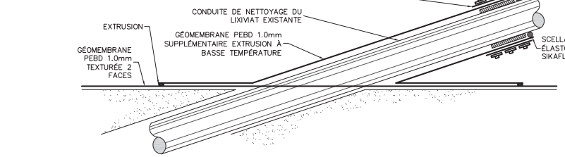
DÉTAIL TIPIQUE MANCHON D'ÉTANCHÉITÉ POUR CONDUITE DE NETTOYAGE Echelle: Aucune
