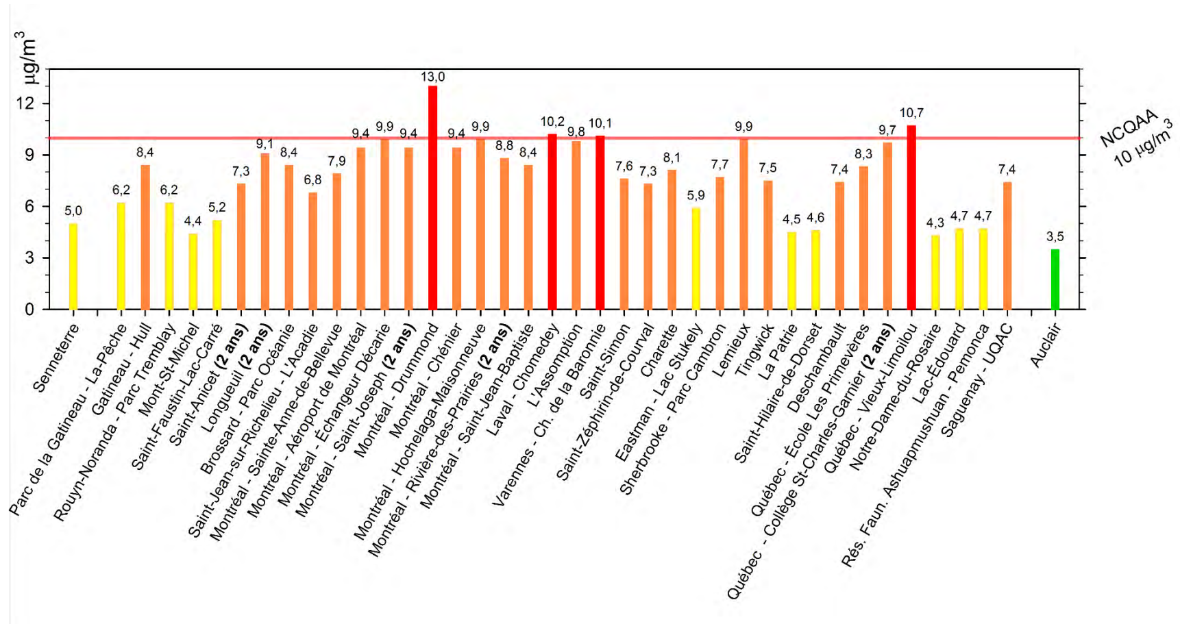
Figure 3 Concentrations de particules fines sous la forme statistique de la NCQAA (année civile) pour la période 2012-2014 Note : (2 ans) indique que la moyenne a été calculée à partir des données de deux années au lieu de trois.
