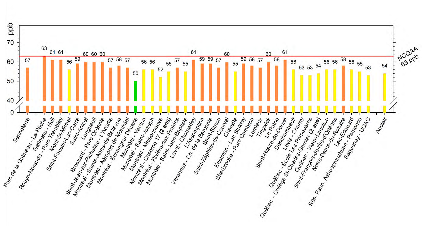
Figure 4 Concentrations d’ozone sous la forme statistique de la NCQAA pour la période 2012-2014
