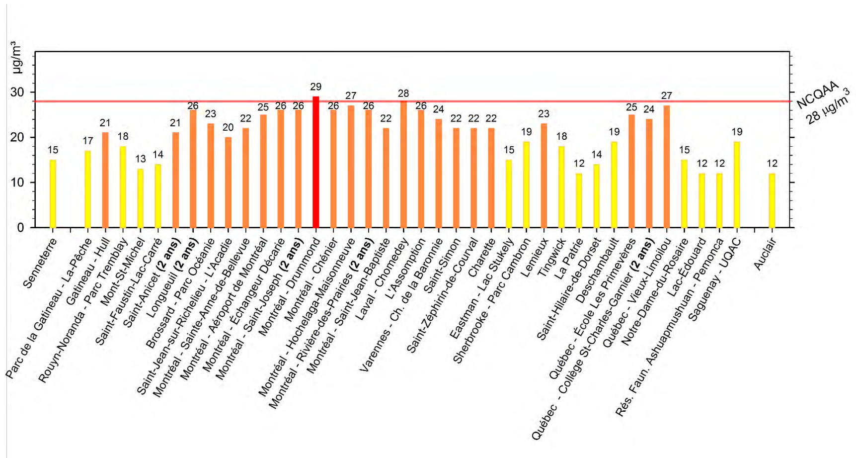
Figure 2 Concentrations de particules fines sous la forme statistique de la NCQAA (24 heures) pour la période 2012-2014 Note : (2 ans) indique que la moyenne a été calculée à partir des données de deux années au lieu de trois.
